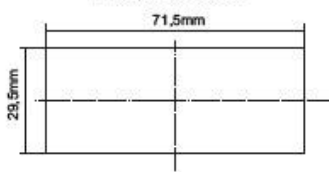
Einbauausschnitt
